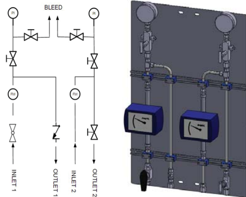
API 682 PLAN 54
